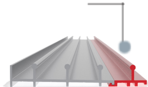
Guía inferior con una extensión.
